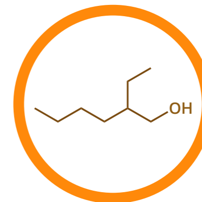
2-ETILHEXANOL
