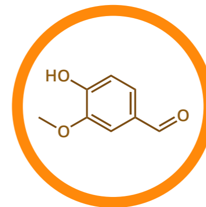
VANIL·LINA
