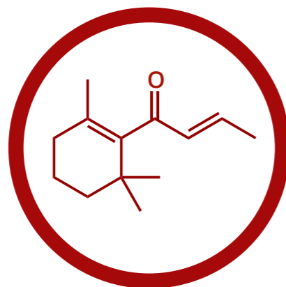
\beta -DAMASCONA
