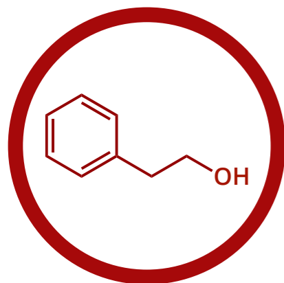
2-FENILETANOL
